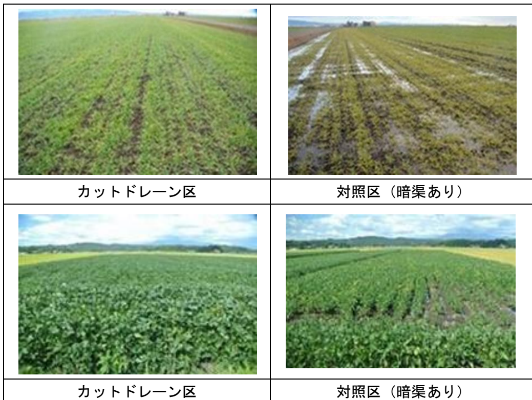
図. カットドレーンの排水性と作物への効果
